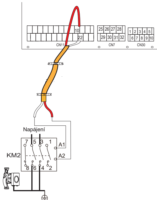
Venkovní oběhové čerpadlo P_o
