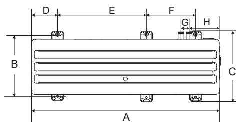
8/10/12/14/16 kW (jednotka: mm)
