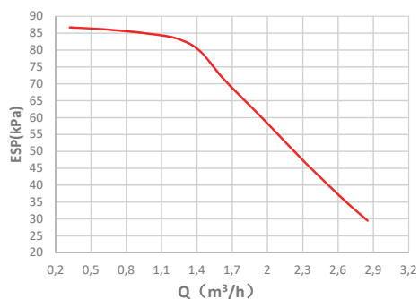
Dostupný externí statický tlak VS Průtok
