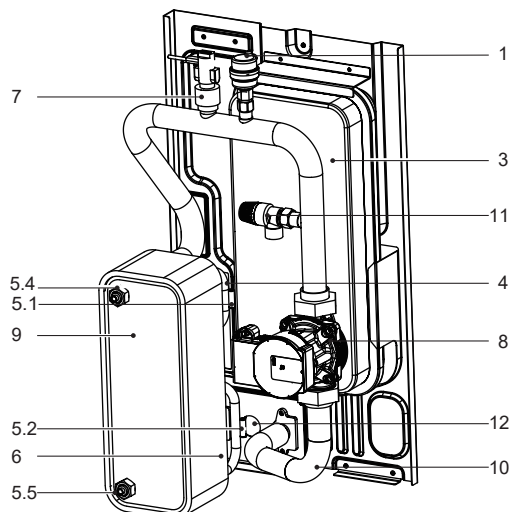
4/6 kW bez záložního ohřívače
