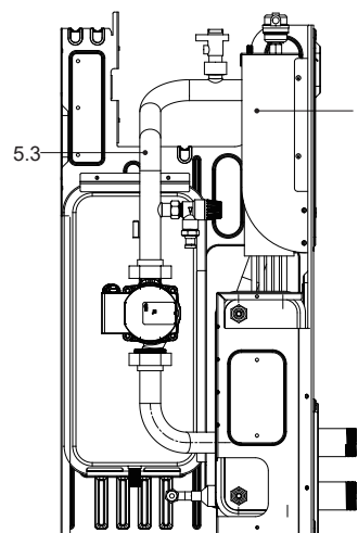
8–16 kW se záložním ohřívačem (volitelné)
