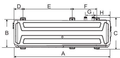
4/6 kW (jednotka: mm)
