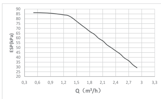
Dostupný externí statický tlak VS Průtok
