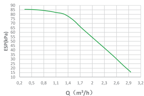
Dostupný externí statický tlak VS Průtok
