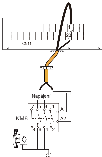
Venkovní solární čerpadlo P_s
