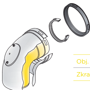
Koleno 90° ø80/125 lité s inspekčním otvorem
